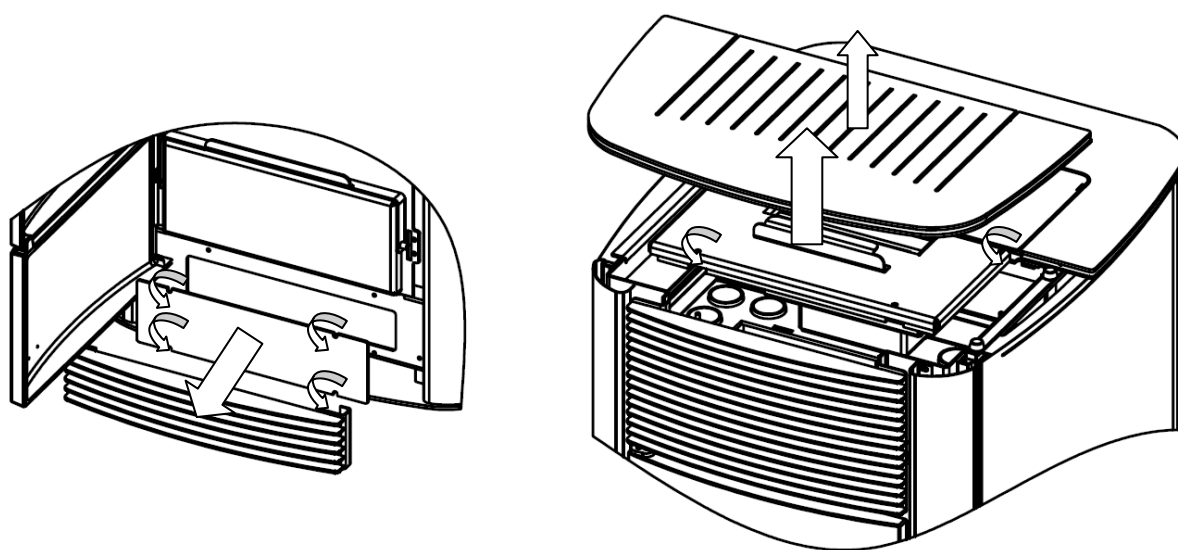
Čišćenje unutrašnjosti peći
